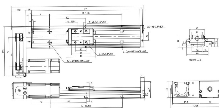
KK60 电机左装
