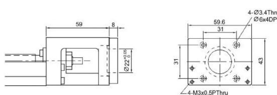
马达连接法兰 F5(42 步进)
