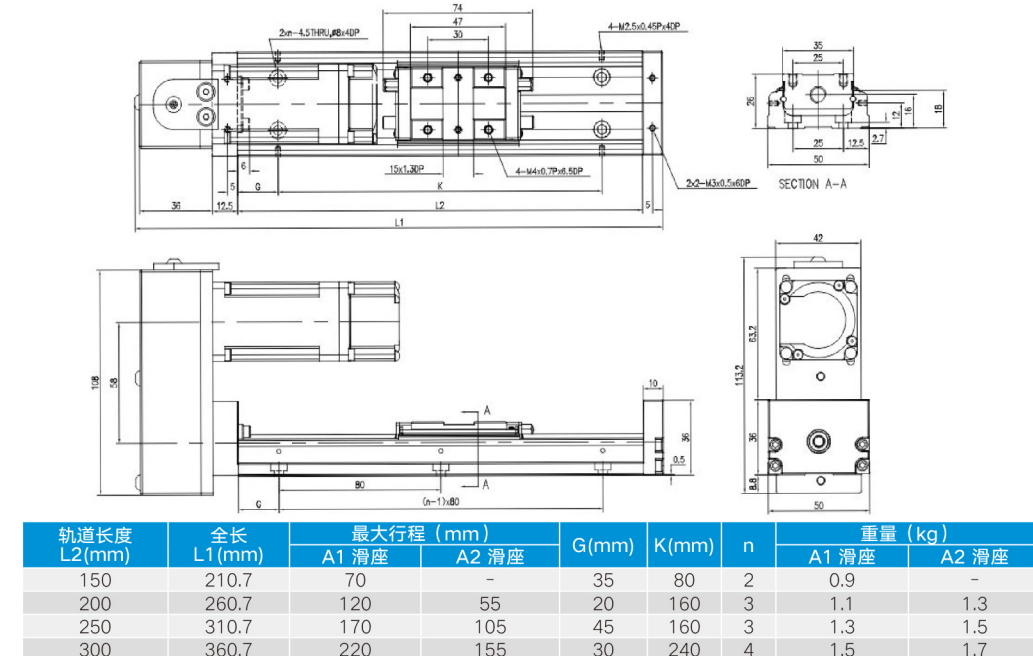
KK50 电机上装
