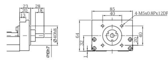
转接固定座 H0( 间接连接 )
