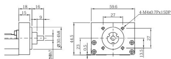
转接固定座 H1( 间接连接、安装孔、与前者不一样 )
