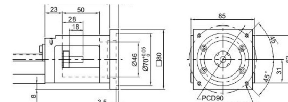
马达连接法兰 F5(60 步进)
