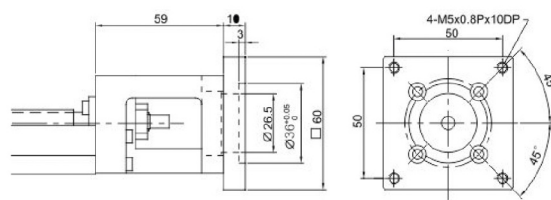
马达连接法兰 F3(60 步进)
