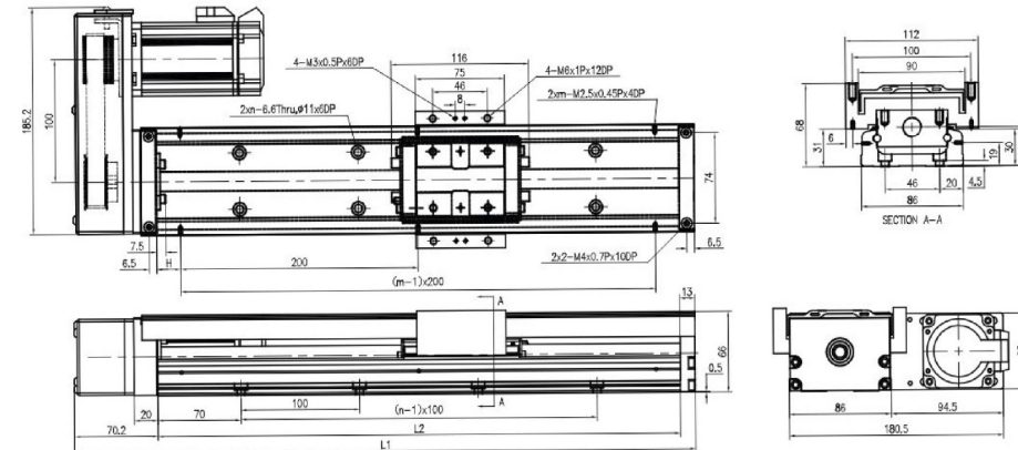
KK86 电机右装
