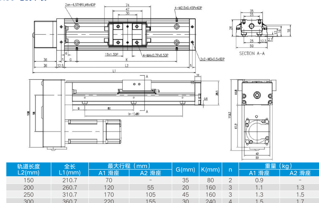
KK50 电机下装
