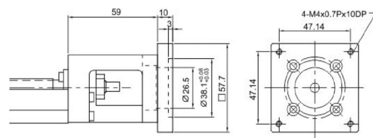
马达连接法兰 F4(57 步进)
