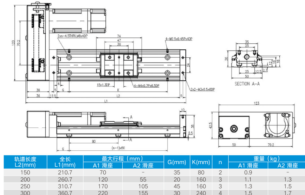
KK50 电机右装
