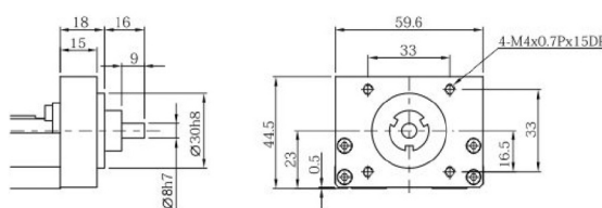
转接固定座 H0( 电机间接连接 )
