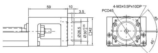
马达连接法兰 F2( 松下 500W、100W)
