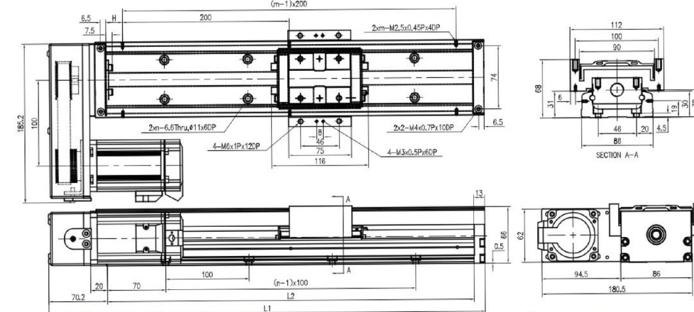
KK86 电机左装
