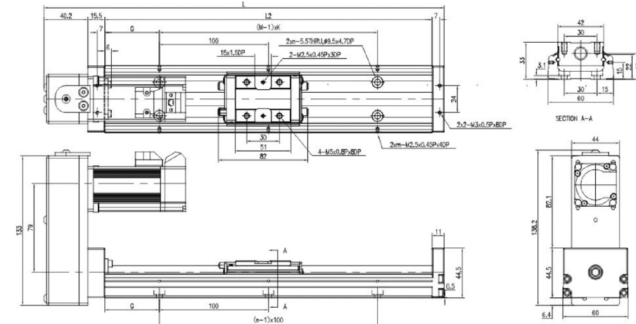
KK60 电机上装
