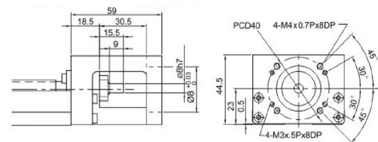
马达座 F0( 无转接法兰 )
